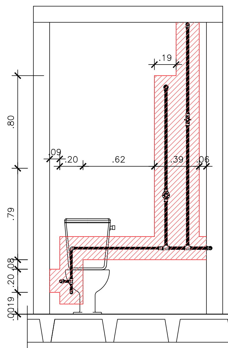
Vista A ESCALA 1/25
