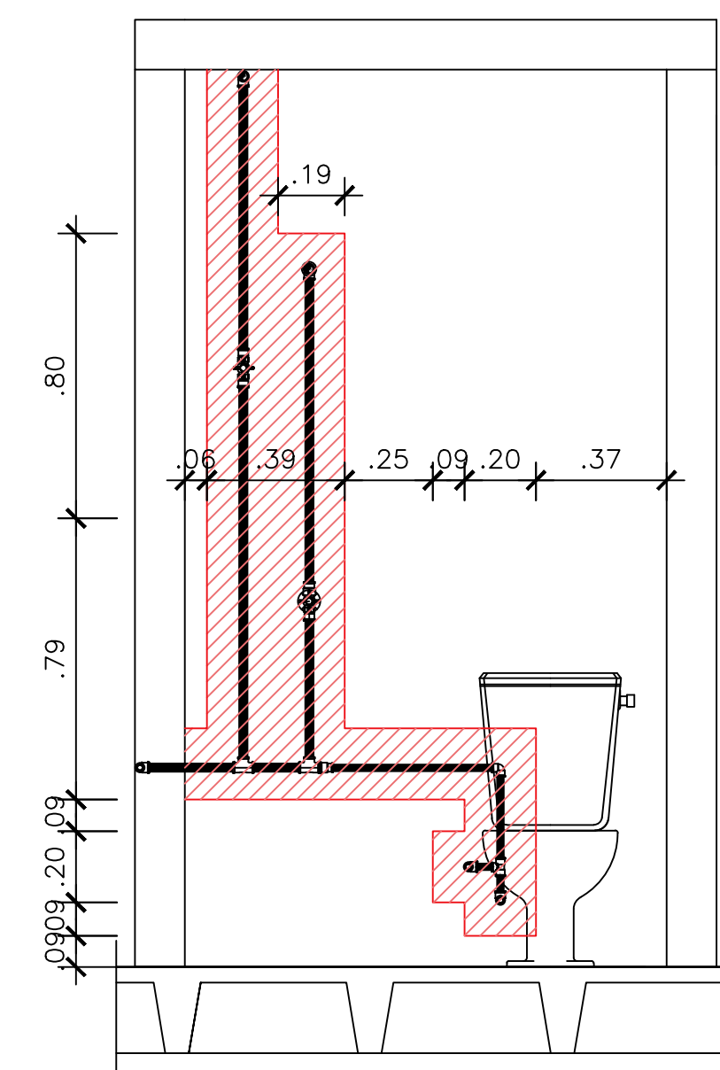
Vista D ESCALA 1/25
